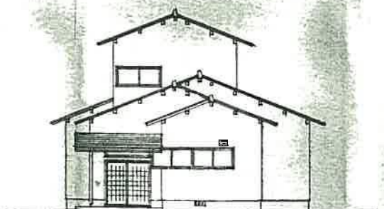
立面图(北) 1:100
