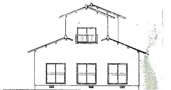
立面图(南) 1:100
