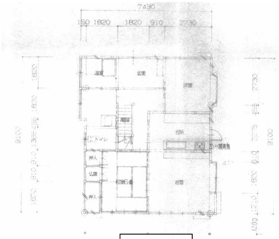
一階平面図
