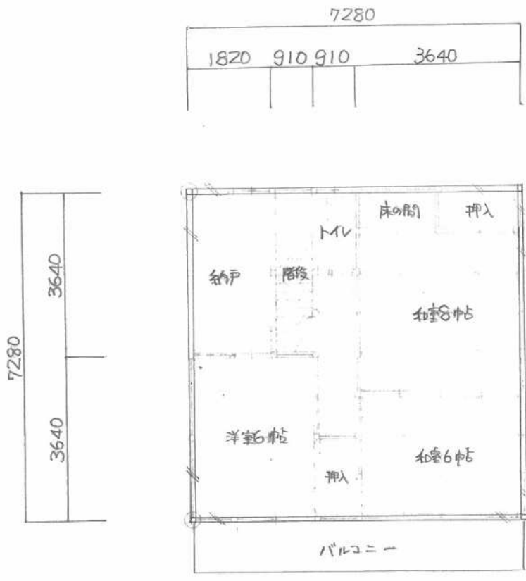
二階平面図
