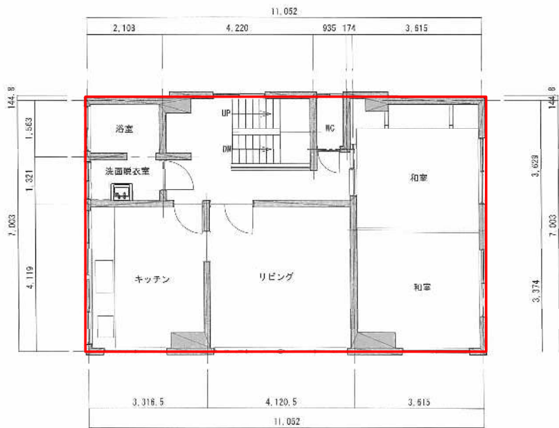
2階平面図
