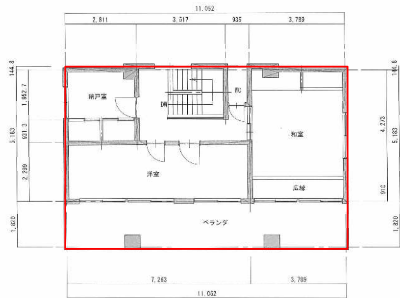
3階平面図
